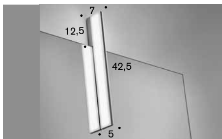
ROSSETTI cromo, possibilità d'installazione verticale o orizzontale IP44 ROSSETTI chrome, vertical or horizontal installation's possibility IP44
