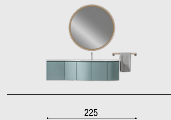
GIU2562 L.225 H.190 P.50 Finiture: Laccato Opaco Denim Top: Stonematt con lavabo Fornace Maniglia: Presa a gola 45° Specchiera: Tonda con cornice — W.225 H.190 D.50 Finish: Matt Lacquered Denim Top: Stonematt with Fornace basin Handle: 45° groove Mirror: Round with frame
