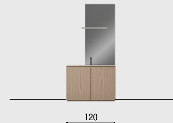
GIU2516 L.120 H.240 P.50 Finiture: Essenza Castagno Cumino Top: Stone Color Agata con lavabo Carena Maniglia: Presa a gola 45° Specchiera: D'arredo Faretto: Kalo Asfalto W.120 H.240 D.50 Finish: Chestnut Essence Cumino Top: Stone Color Agata with Carena basin Handle: 45° groove Mirror: Decorating mirror Spotlight: Kalo Asfalto
