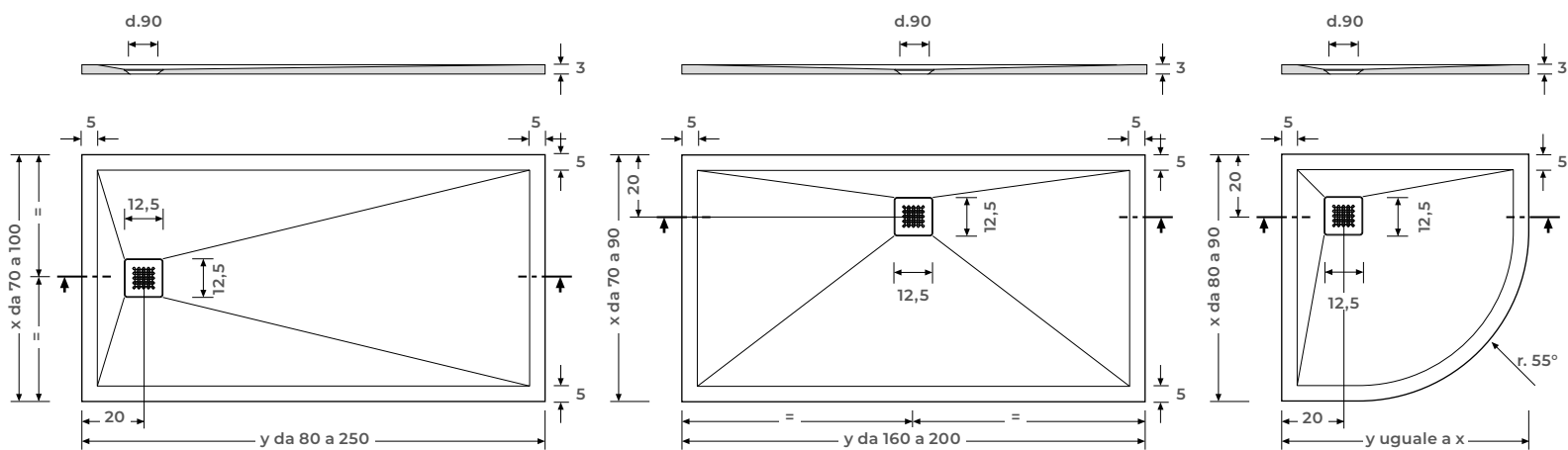
SCARICO LATERALE Lateral Drain
