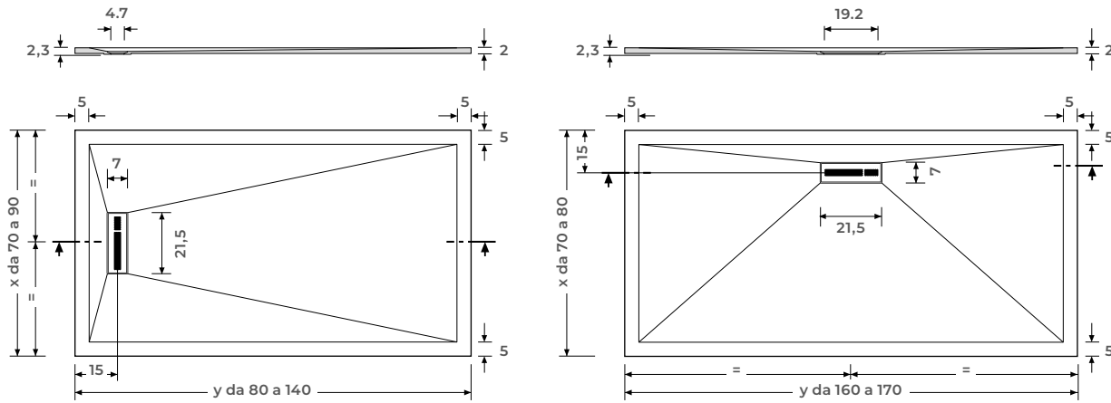
SCARICO LATERALE Lateral Drain
