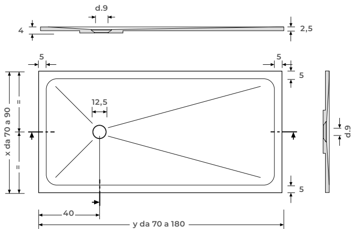
SCARICO LATERALE Lateral Drain
